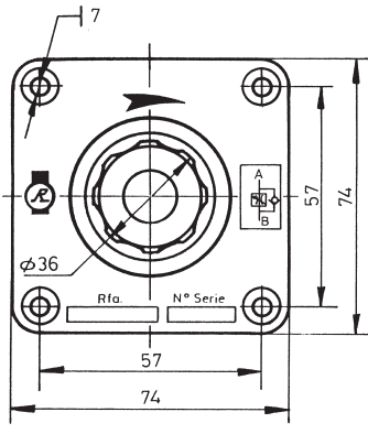
▲ Regulación forma Adjusting type 4
