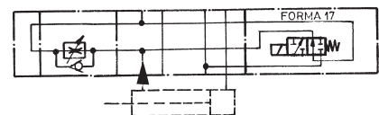
VARIANTE 2: Regulación por "A" en la entrada. Velocidad rápida. VERSION 2: Fast meter out.
