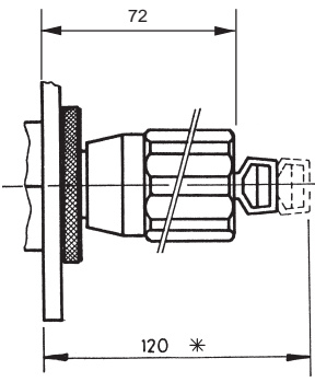
▲ Regulación forma Adjusting type 4
