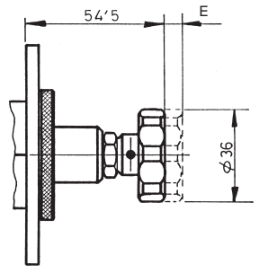
▲ Regulación forma Adjusting type 1
