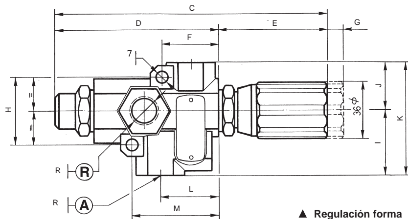
▲ Regulación forma 3 Adjusting type
