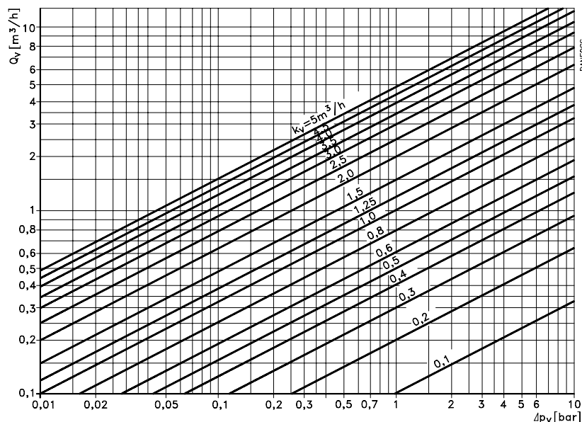
Fig. 2 Relación entre la cantidad de agua y la caída de presión en la válvula. Ejemplo: Caudal de 0,85\text{ m}^3/\text{h} con una caída de presión de 1,5 bar. El valor k_v se convierte en 0,7\text{ m}^3/\text{h} .
